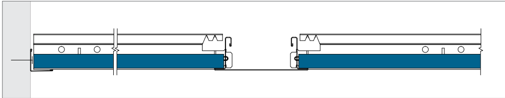
Finition périphérique avec cornière de rive.
