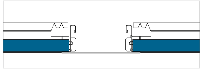
Coupe dalle bord A et porteur de lisse plate.
