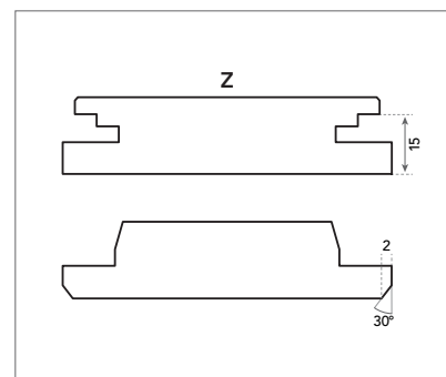
Détails du bord Z : Bord Z1 crée une ligne droite dans une direction, alors que le bord Z2 dissimule l'ossature.
